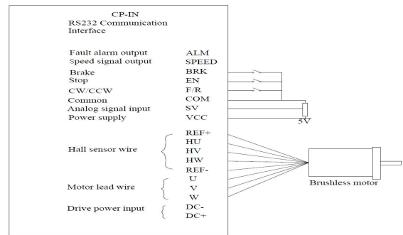
BLDC-5025A
